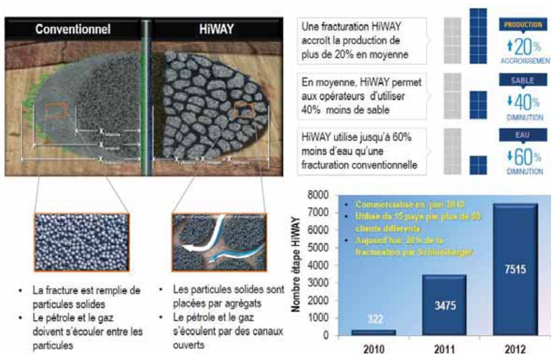
HiWAY : EXEMPLE D'UNE NOUVELLE TECHNOLOGIE DE FRACTURATION HYDRAULIQUE
