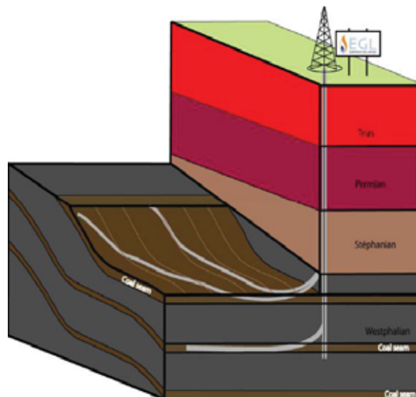
PRINCIPE DU FORAGE HORIZONTAL MULTILATÉRAL POUR L'EXTRACTION DU GAZ DE HOUILLE
